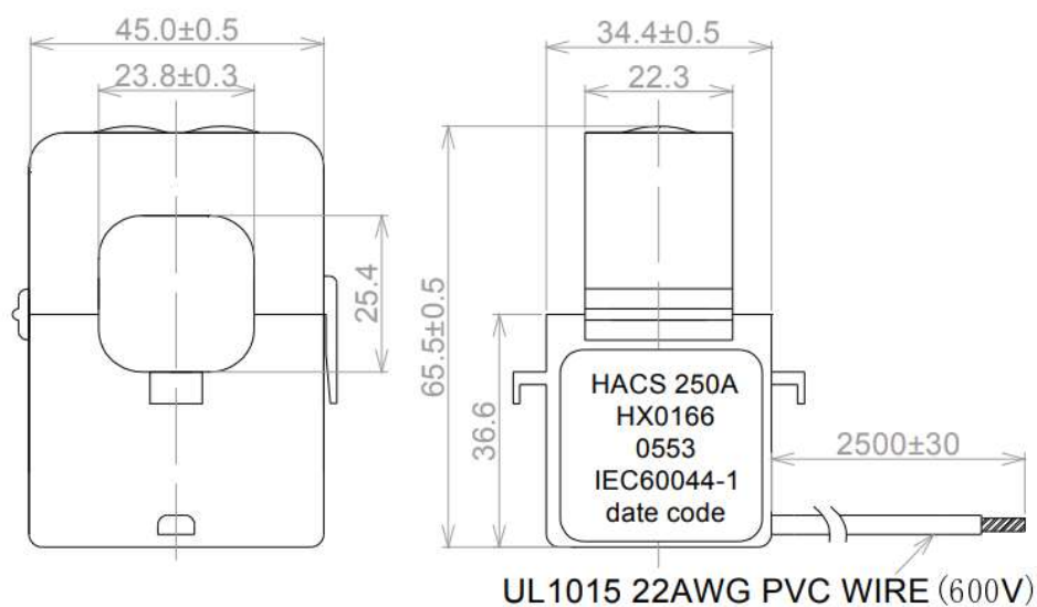
Рисунок 21 – Размеры трансформатора модификации CS2.5S
