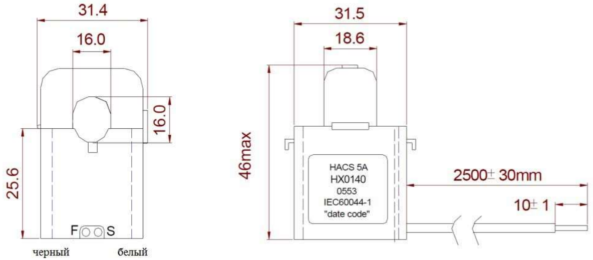
Рисунок 8 – Размеры трансформатора модификации CS05S
