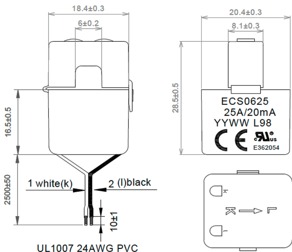
Рисунок 20 – Размеры трансформатора модификаций CS025S, CS03S (25 А)
