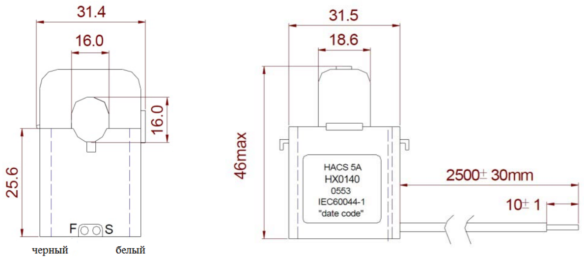
Рисунок 8 – Размеры трансформатора модификации CS05S
