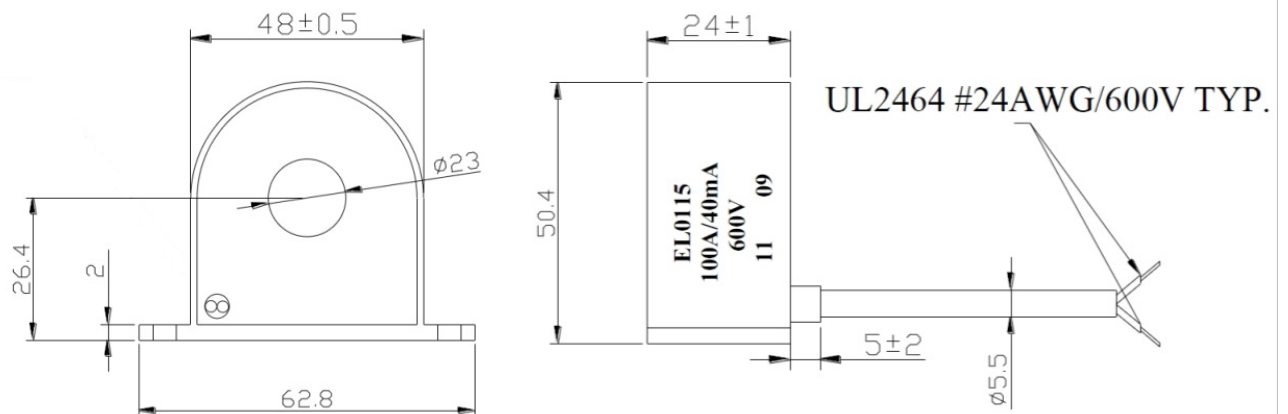
Рисунок 10 – Размеры трансформатора модификации CS1L
