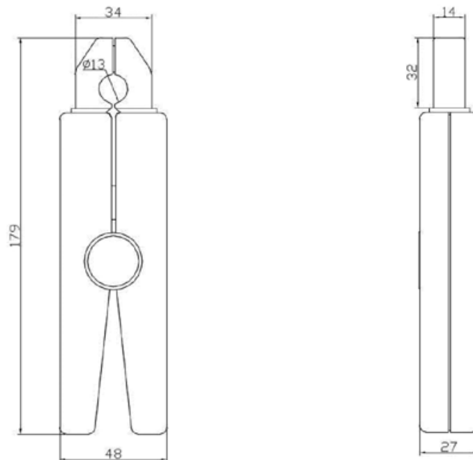
Рисунок 12 – Размеры трансформатора модификации CS1H
