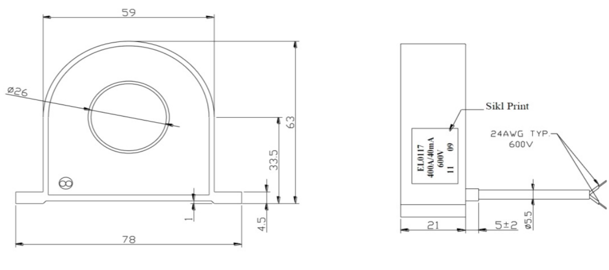
Рисунок 16 – Размеры трансформатора модификации CS4
