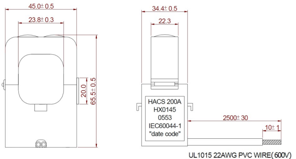
Рисунок 14 – Размеры трансформатора модификации CS2S
