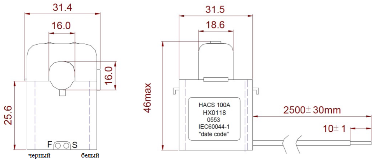
Рисунок 11 – Размеры трансформатора модификации CS1S
