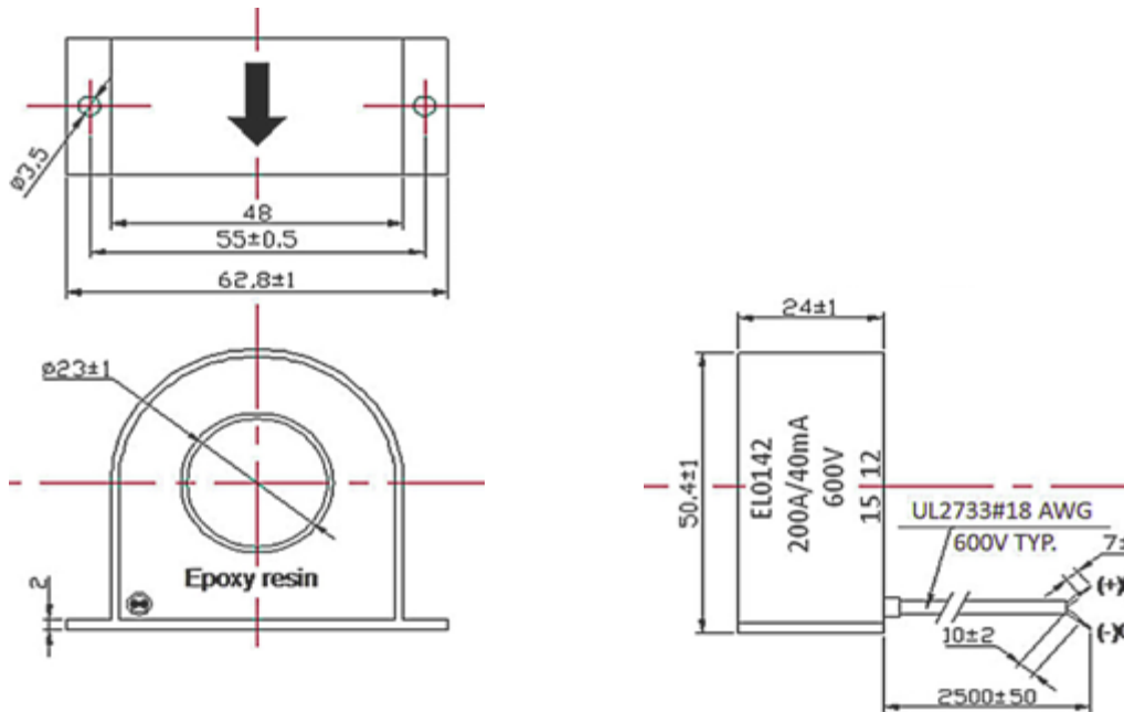
Рисунок 13 – Размеры трансформатора модификации CS2
