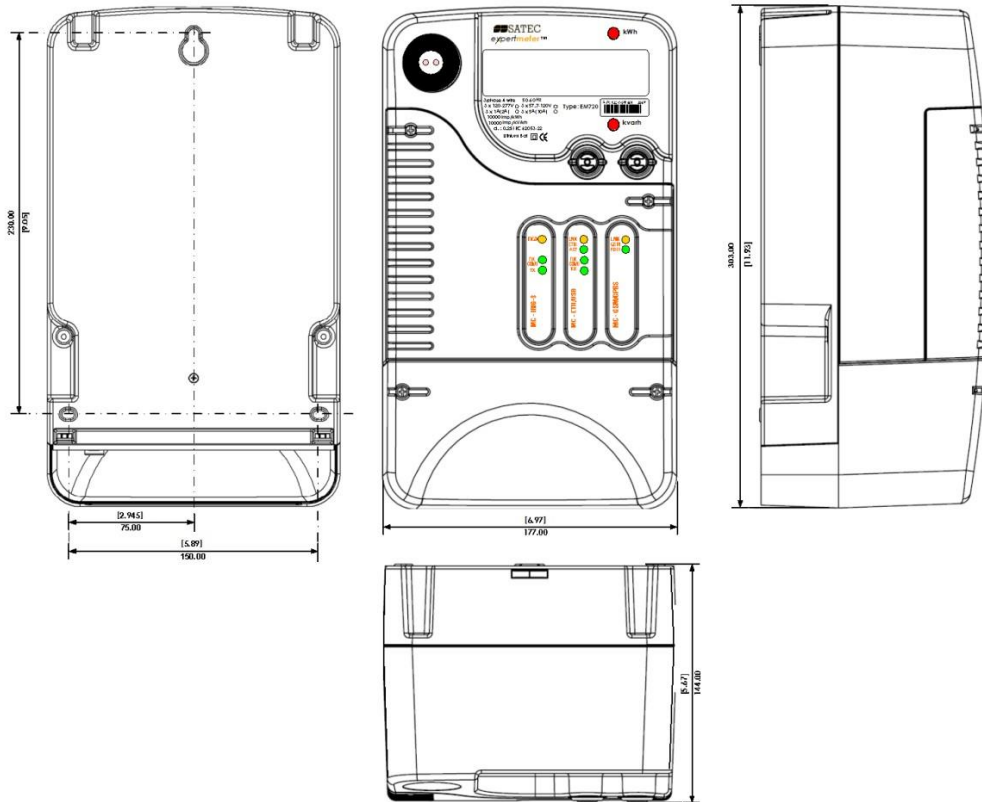
Рис.1 Размеры прибора
