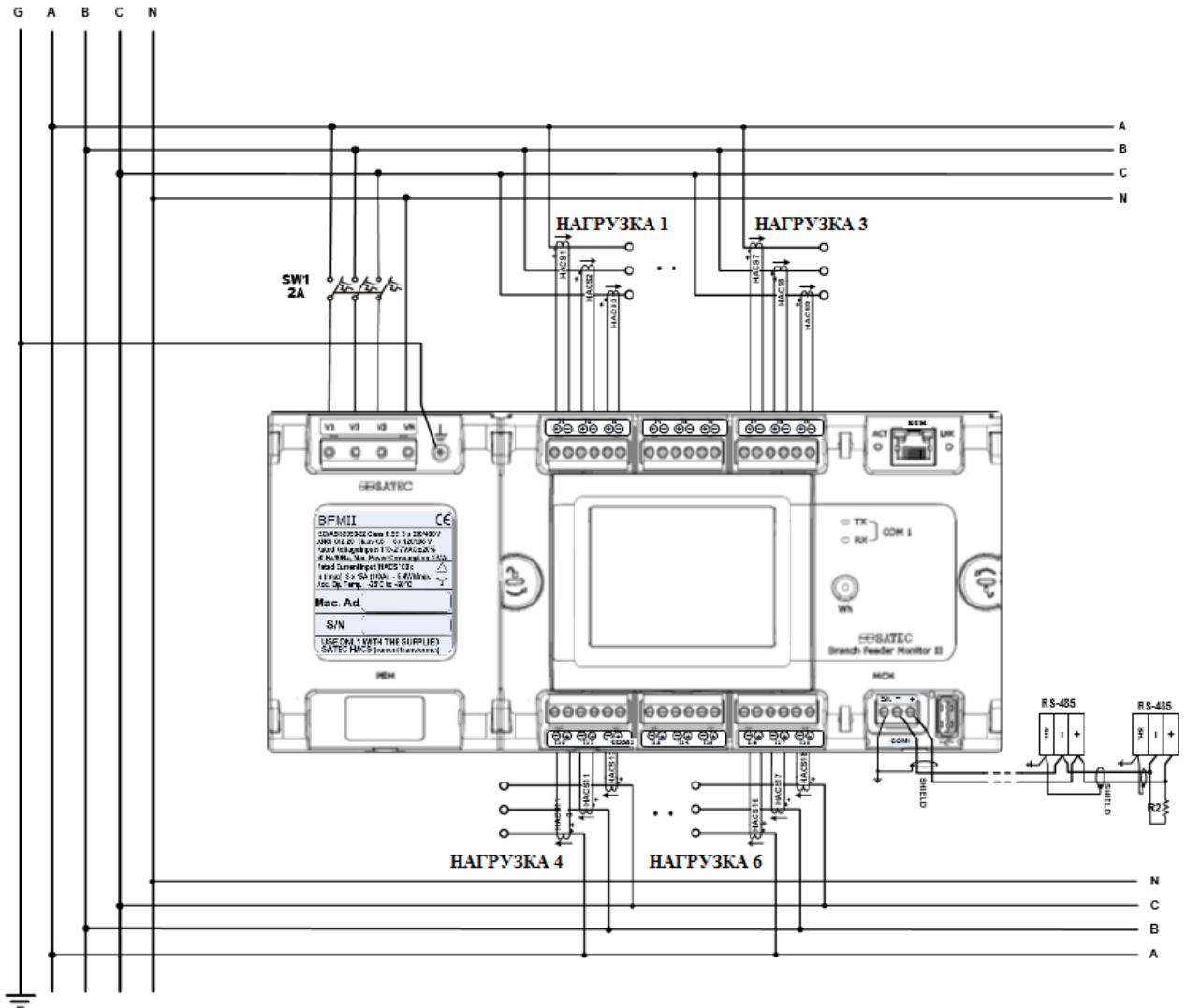
Рисунок 18 – Соединение 4LN3
