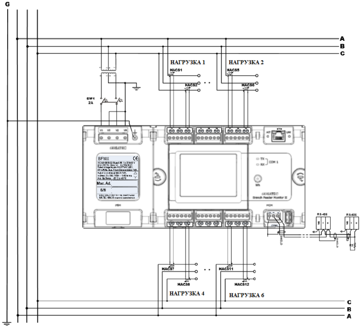
Рисунок 20 – Соединение 3ØP2
