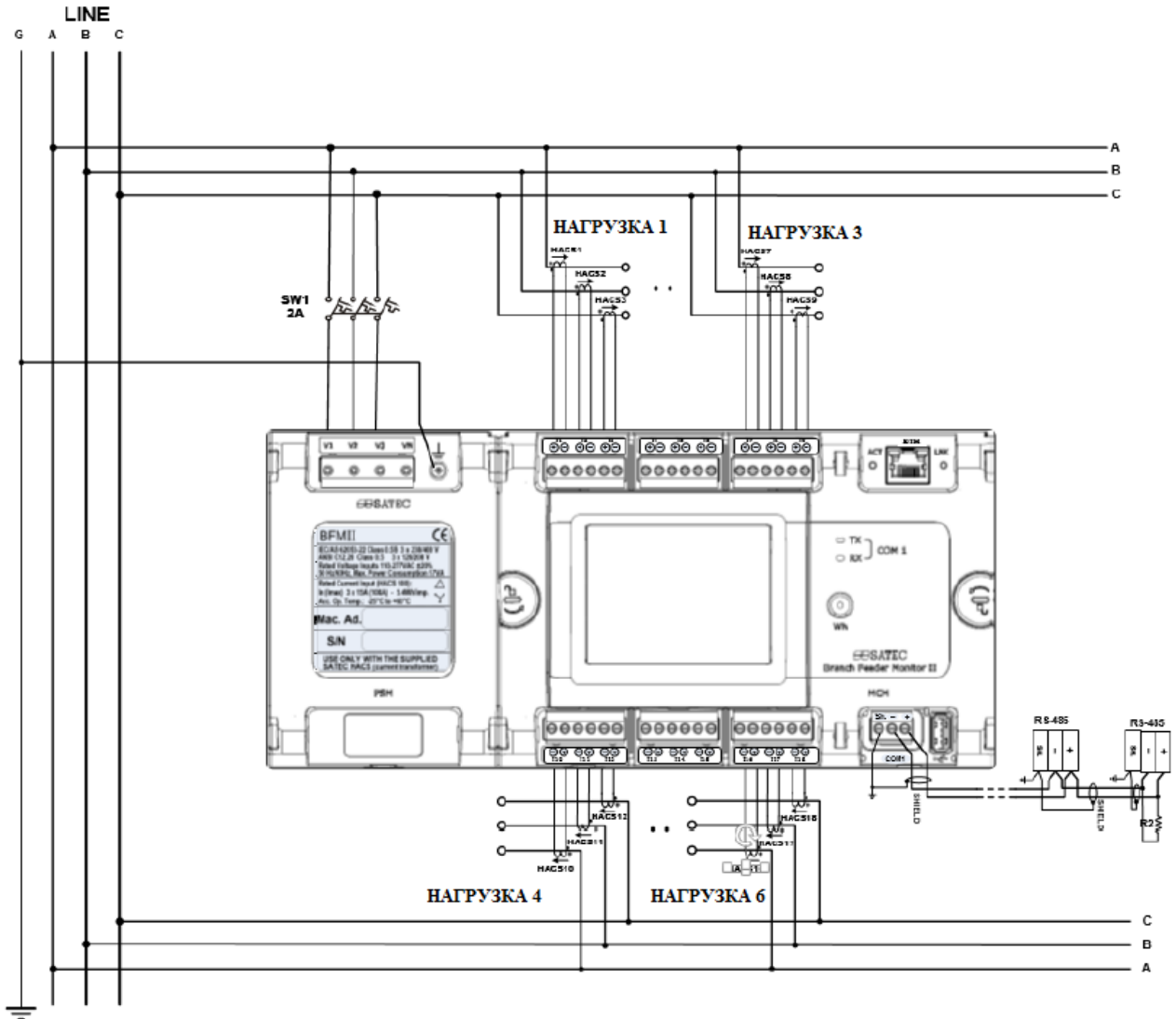
Рисунок 19 – Соединение 4LL3
