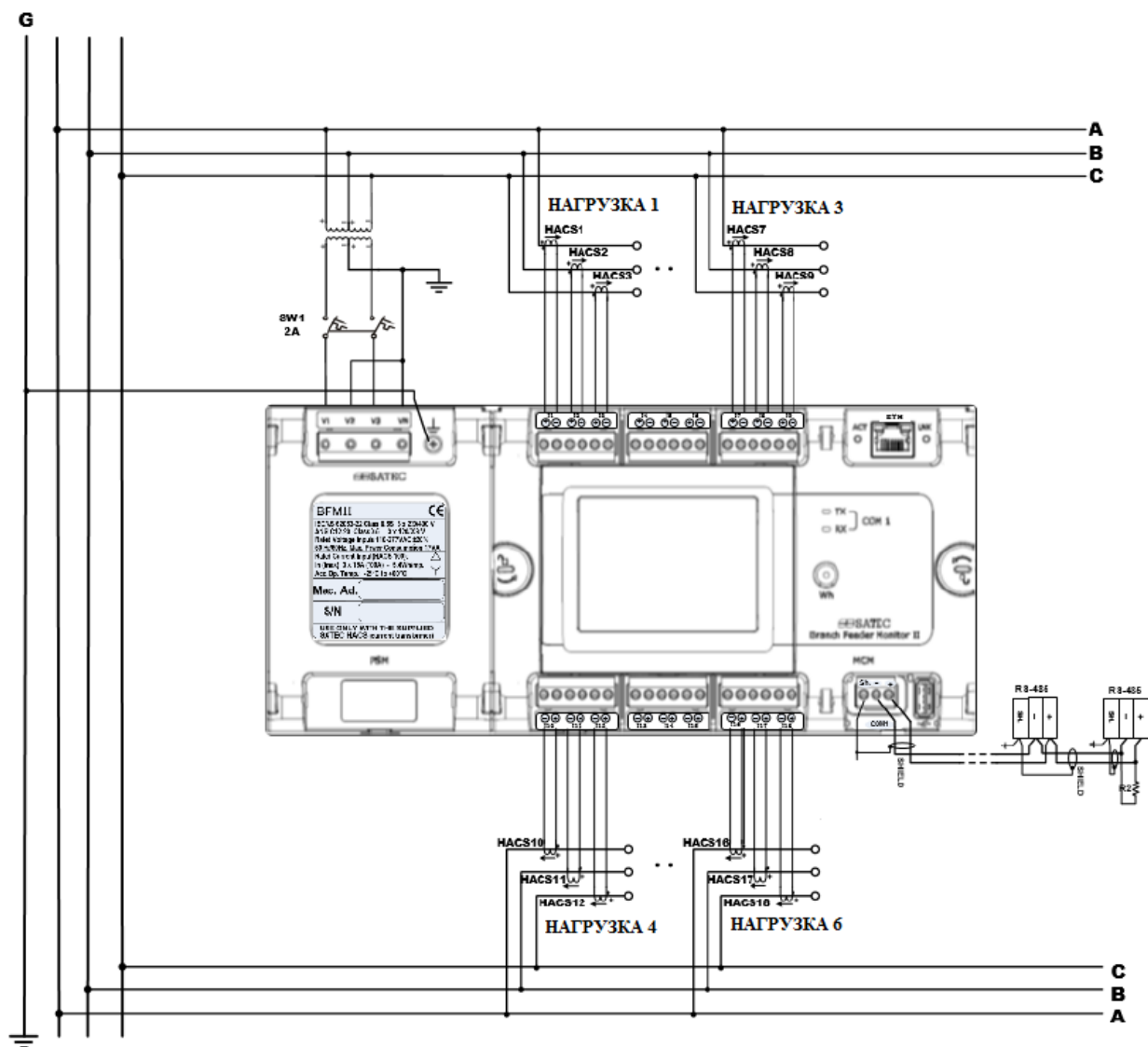
Рисунок 21 – Соединение ЗОРЗ
