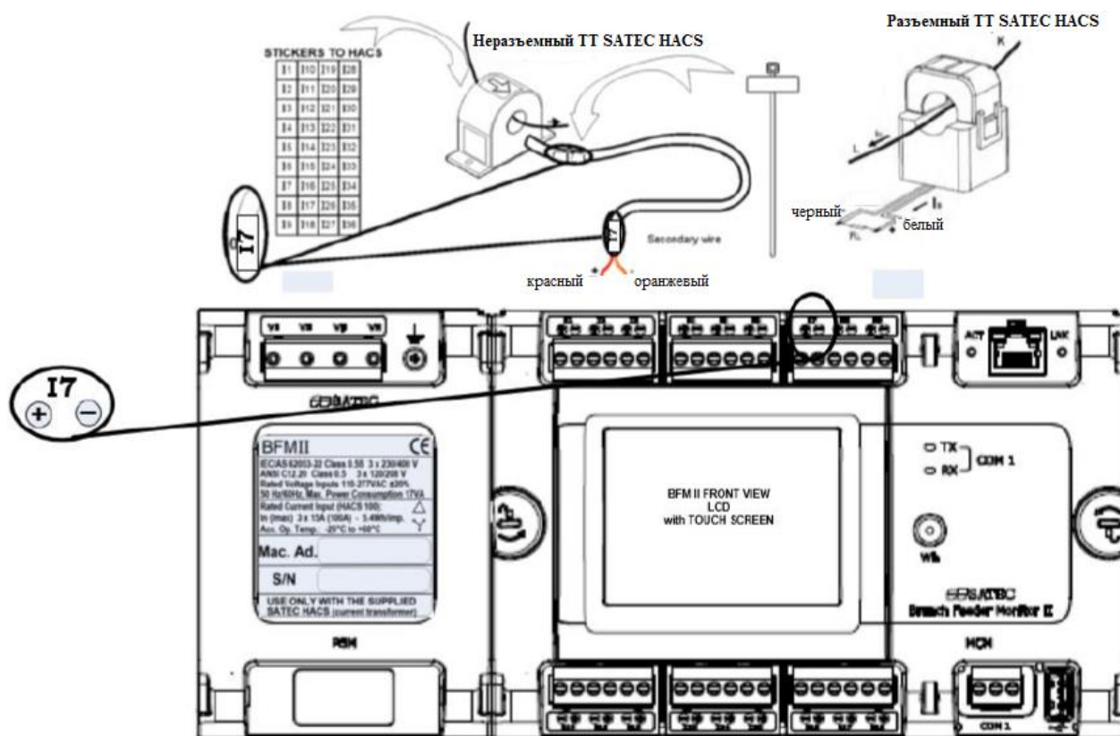
Рисунок 24 – Схема подключения трансформаторов тока SATEC HACS
