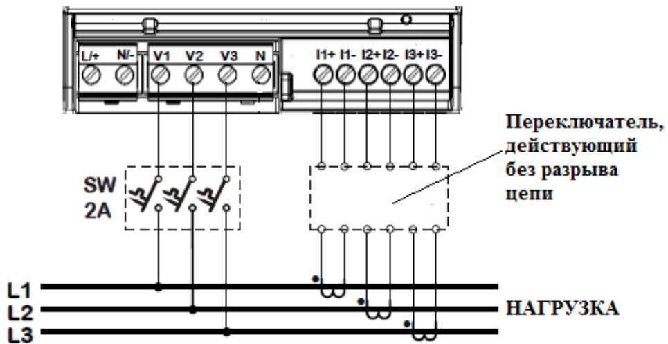
Рисунок 20 – Трёхпроводное трёхэлементное соединение треугольником с использованием 3 ТТ (код настройки 4LL3)
